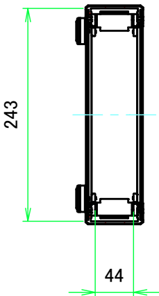
A-A ( 1:6 )
