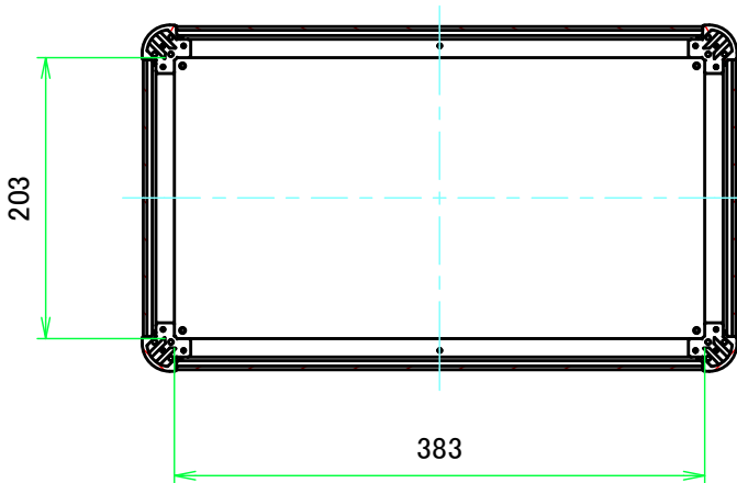
C-C ( 1:6 )
