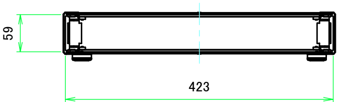
B-B ( 1:6 )
